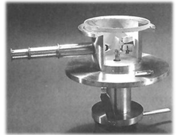
Модель установки Гейгера-Мардсена
