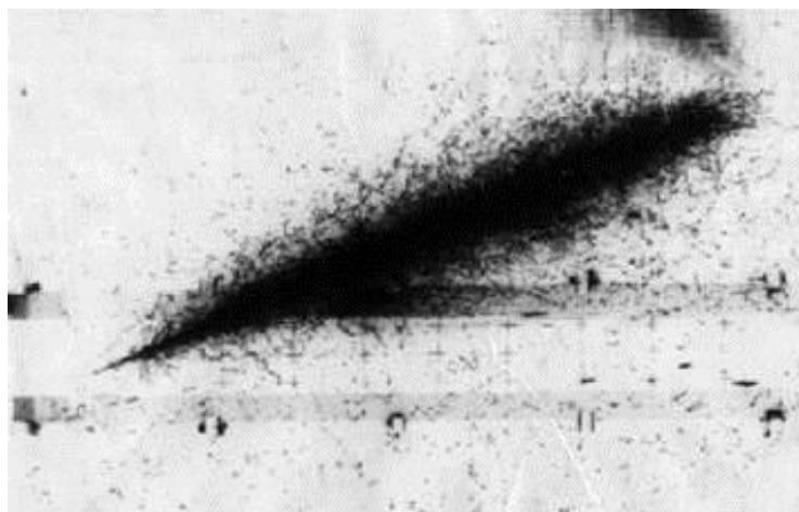
Фотография электромагнитного ливня в 180-литровой ксероновой камере ИТЭФа
